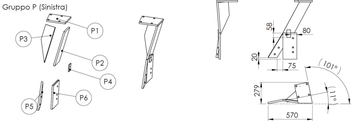
Figura 7. Dispositivi di attacco posteriori
