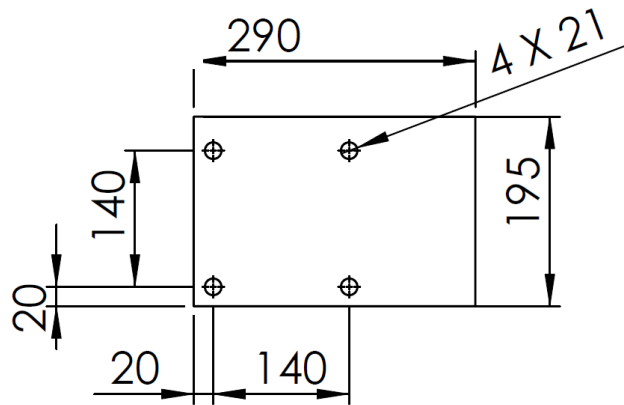
Figura 19. Elemento A4
