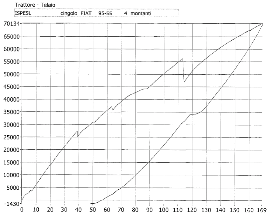
Figura 23. Spinta laterale sinistra
