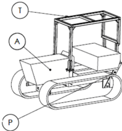
Figura 22. Struttura di protezione per trattori a cingoli modello Fiat 955 e simili
