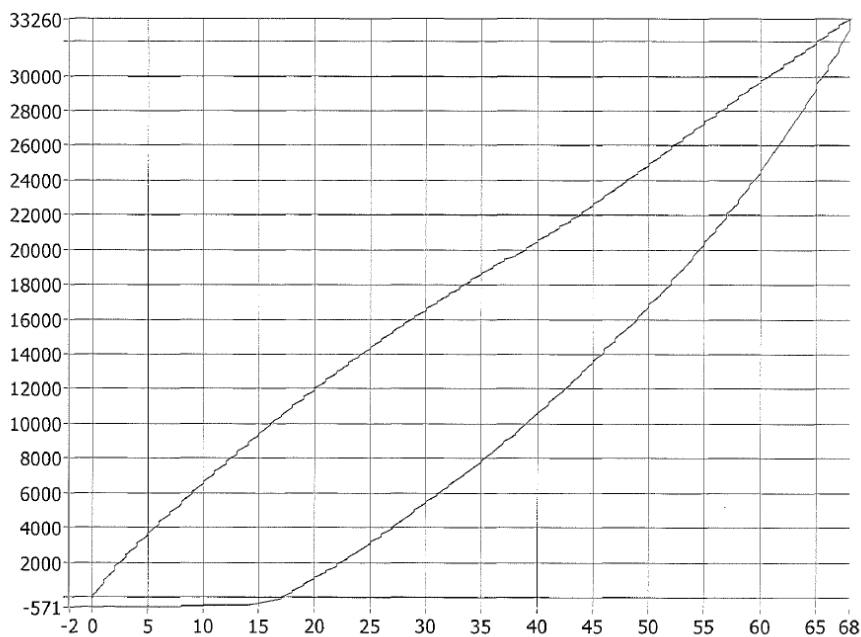
Figura 26. Spinta longitudinale posteriore
