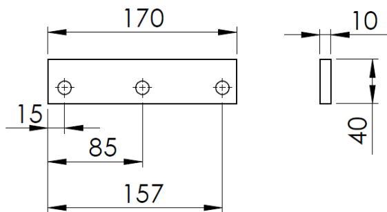
Figura 11. Elemento A9
