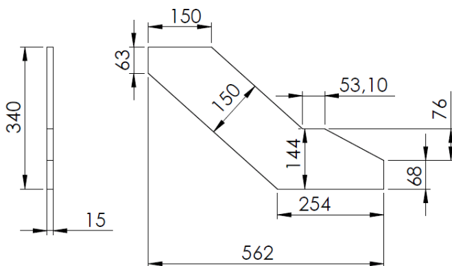
Figura 4. Elemento A2
