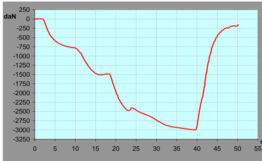
Figura 22. Secondo schiacciamento
