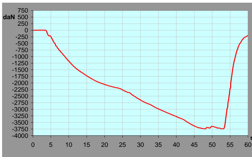
Figura 15. Primo schiacciamento
