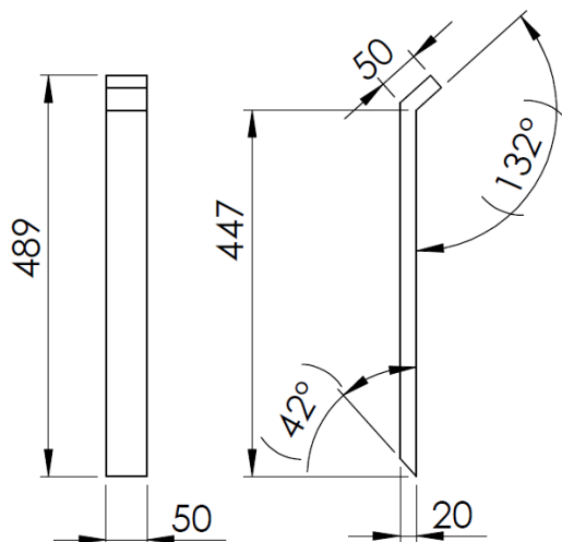
Figura 8. Elemento A6
