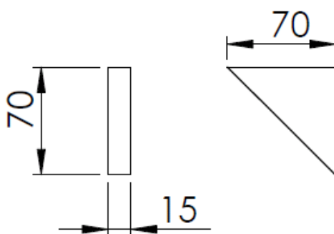
Figura 7. Elemento A5
