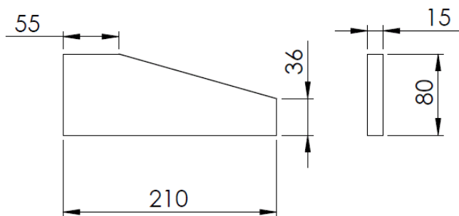
Figura 6. Elemento A4
