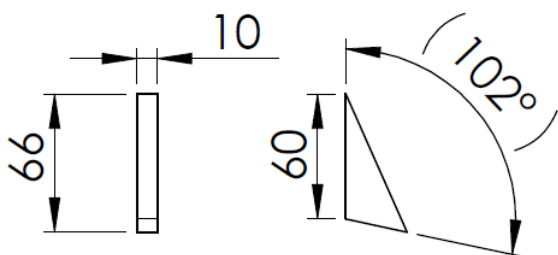
Figura 12. Elemento A10
