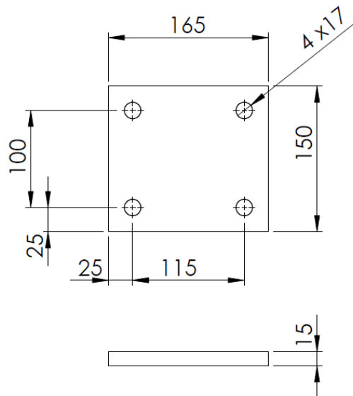
Figura 3. Elemento A1
