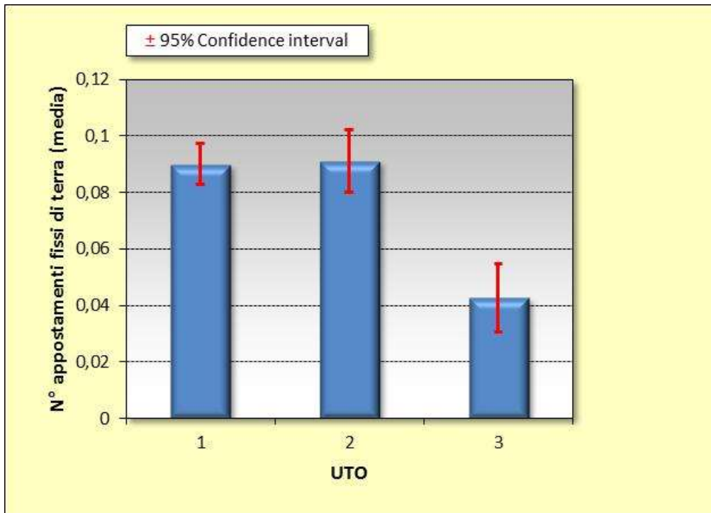
1.10.2-F4 Distribuzione media delle variabili (alcune accorpate) incluse nella AFD tra le UTO.
