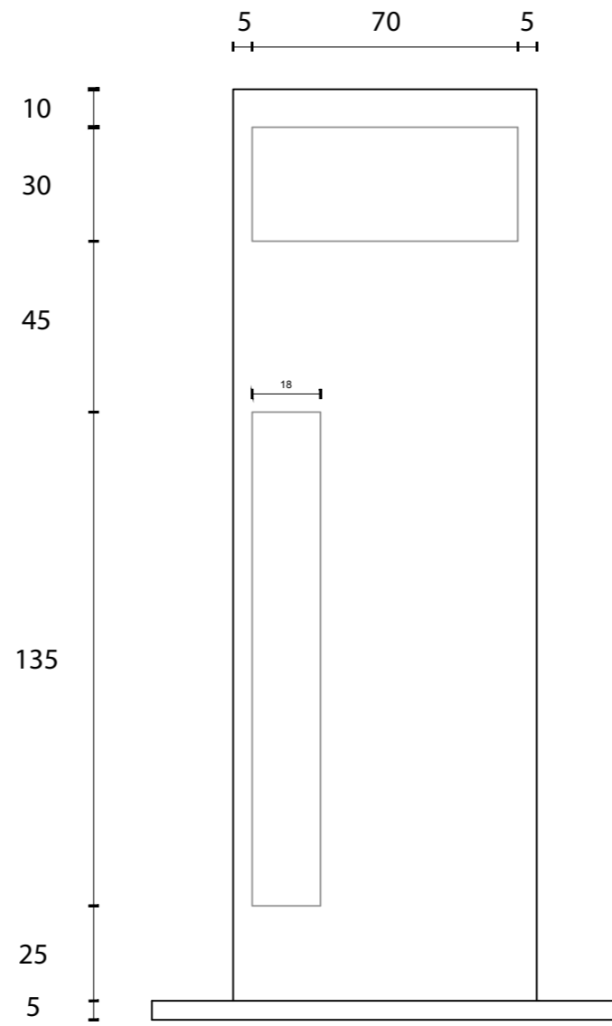
prospetto frontale
