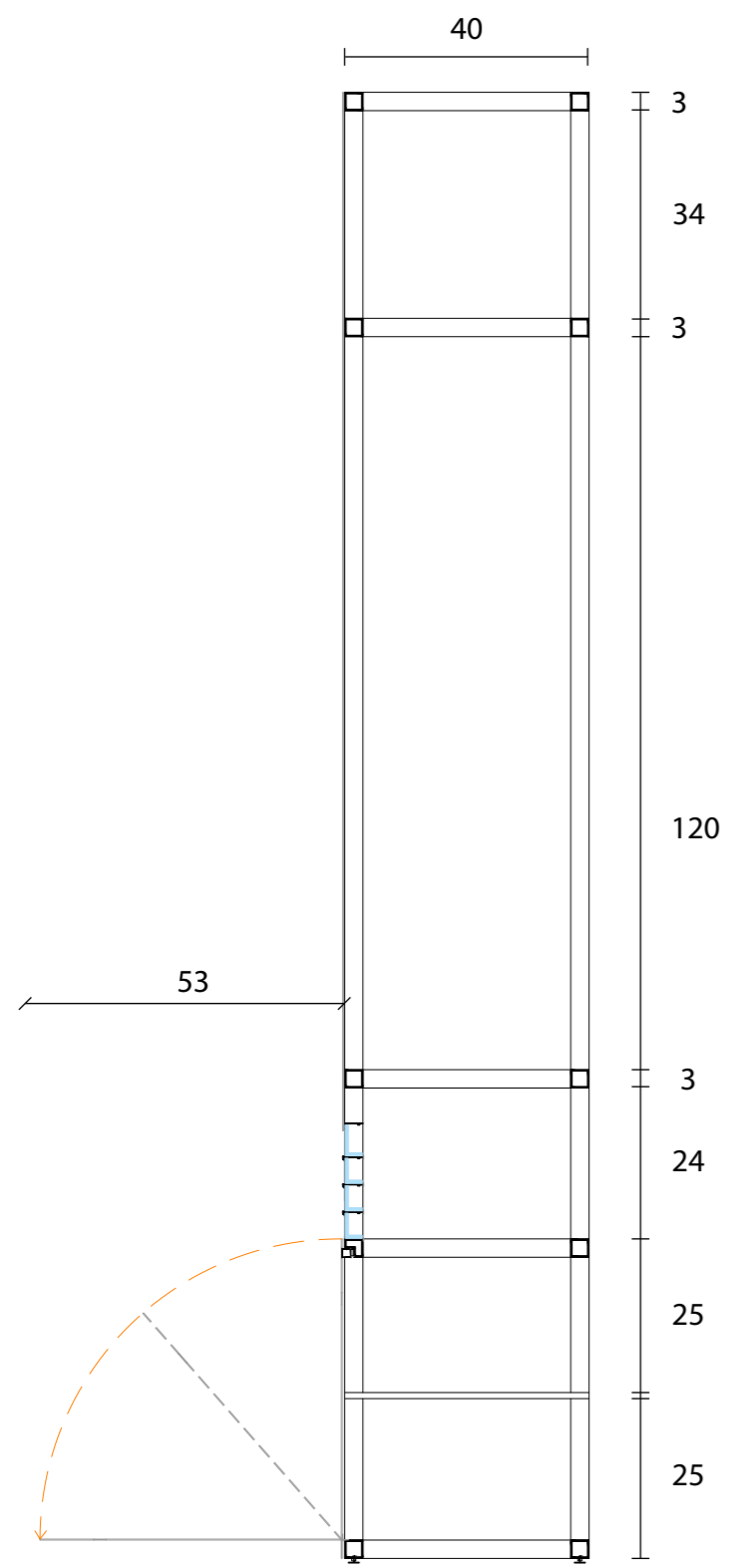
sezione trasversale
