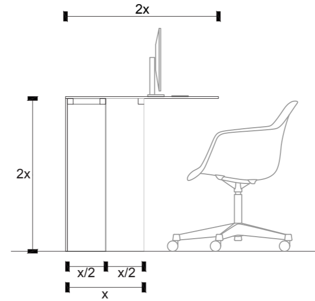
sezione trasversale
