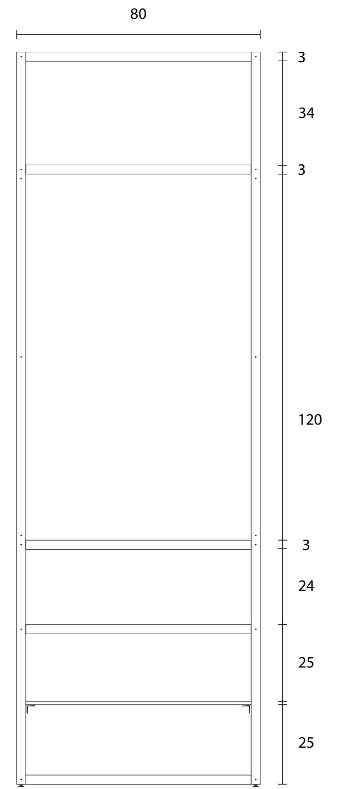
sezione longitudinale
