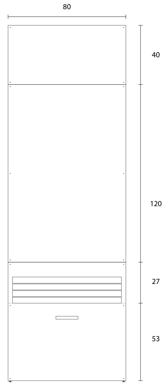
prospetto
