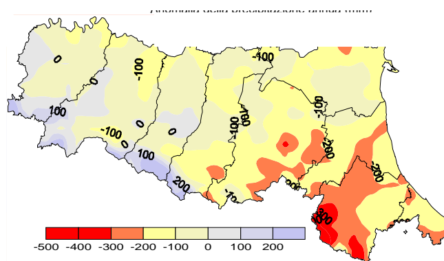
Figura 13 Anomalia delle precipitazioni annuali del periodo 2006-2008 rispetto al quindicennio 1991-2005
